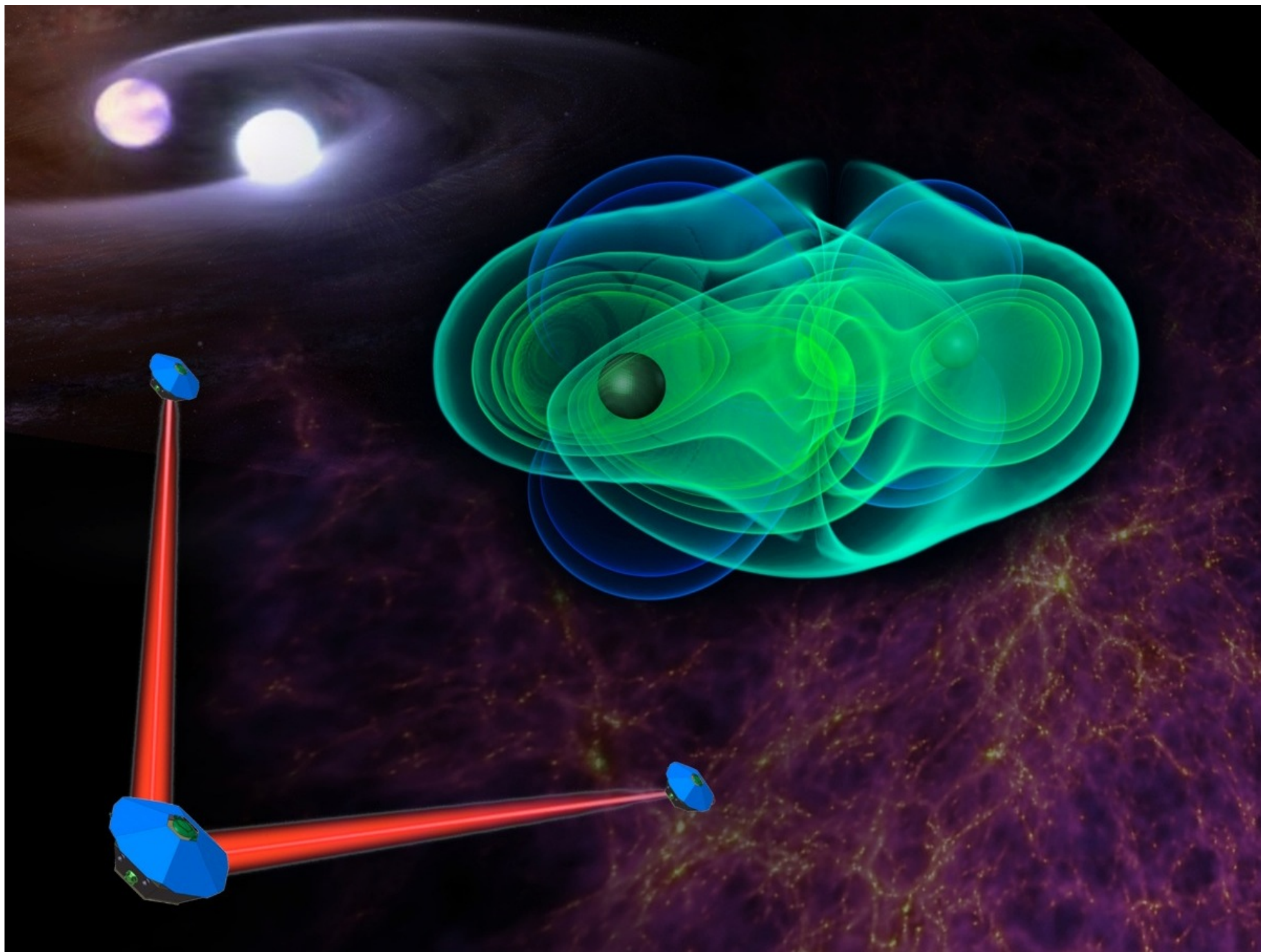
eLISA/NGO
