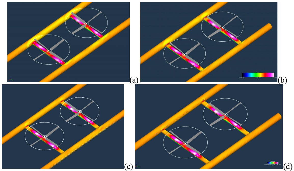
Figure 21. Wing upper-surface pressures: (a) b/R=2.09 ; (b) 2.46; (c) 2.71; (d) b/R=2.95
