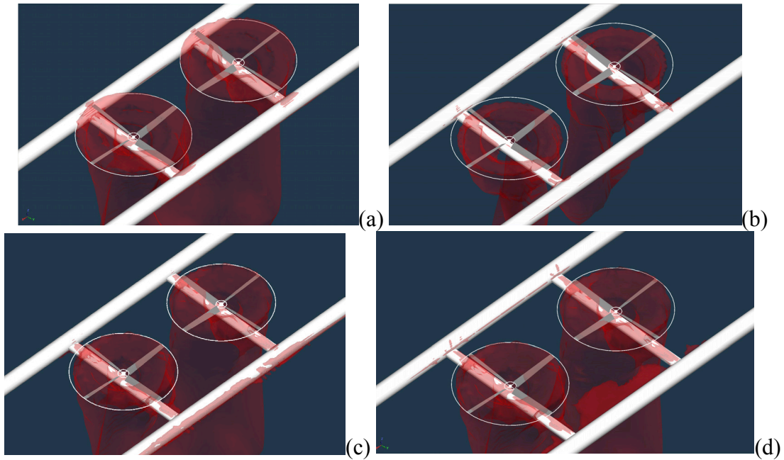
Figure 20. Rotor wake velocity magnitude isosurfaces: (a) b/R=2.09 ; (b) 2.46; (c) 2.71; (d) b/R=2.95
