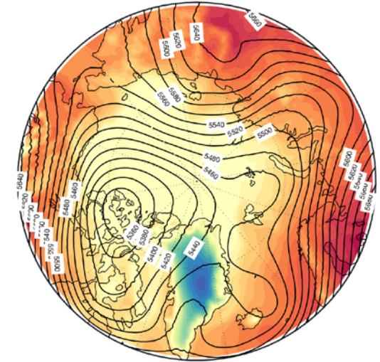
MERRA-2
