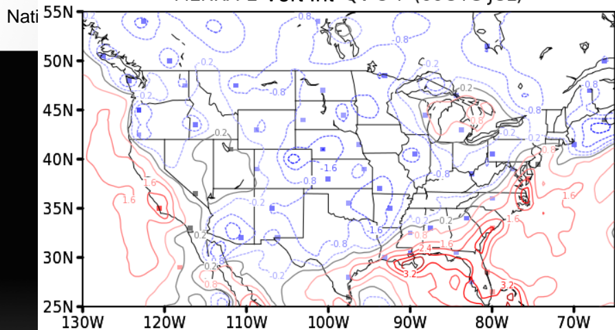
MERRA-2 Vert Int Qv O-F (00UTC JUL)
