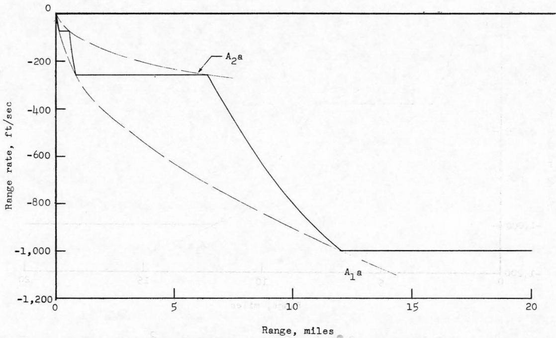
(d) A_1a = 8 \text{ ft/sec}^2 ; A_2a = 1 \text{ ft/sec}^2 .
