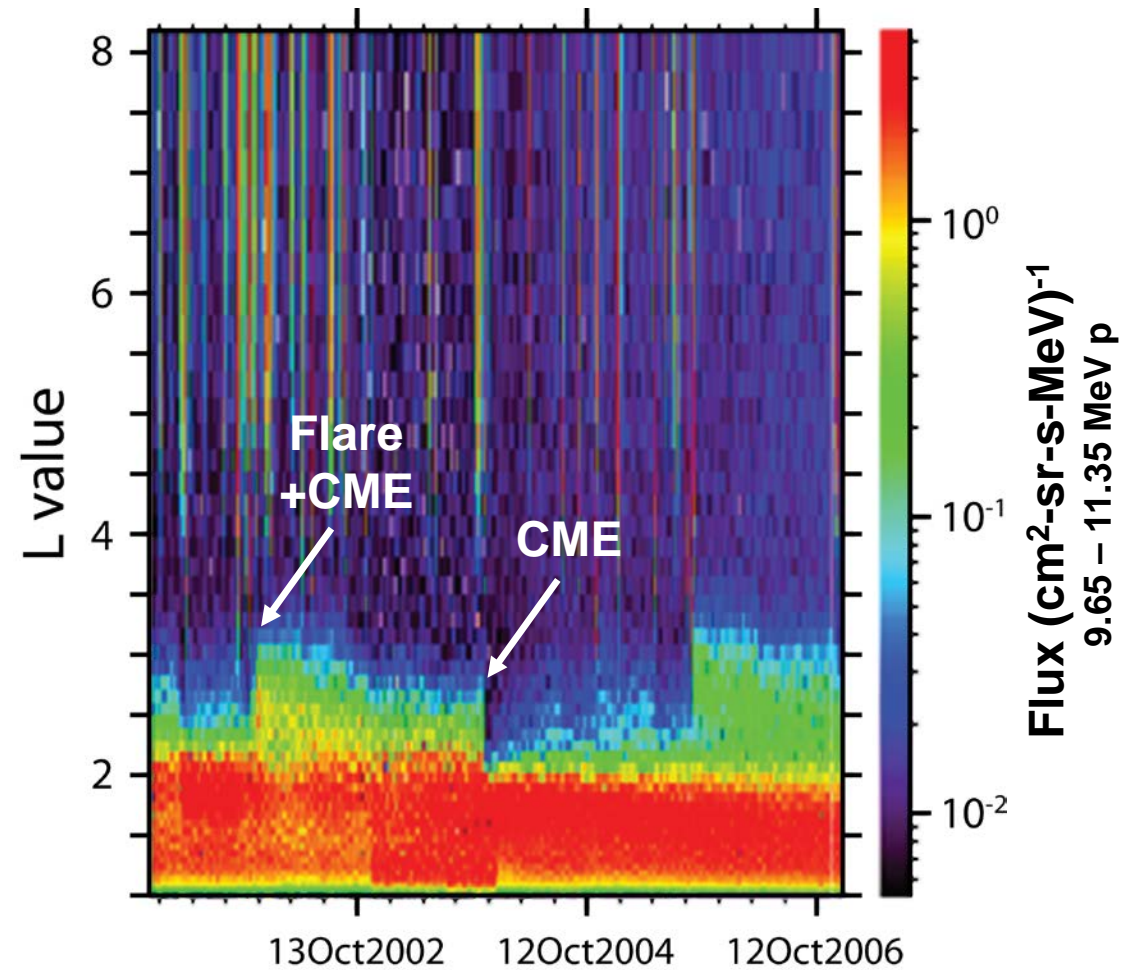
S. Bourdarie and M.A. Xapsos, IEEE TNS, Aug. 2008
