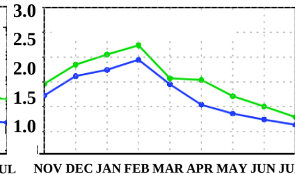
T 2m , Europe
