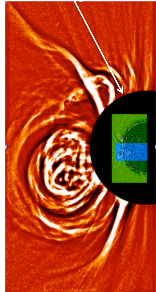
LASCO-C2+SWAP+AIA
