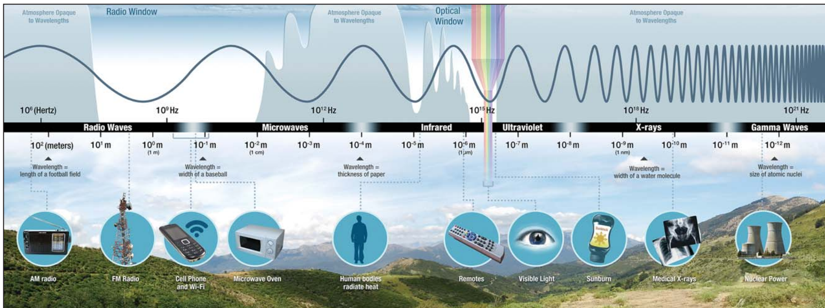
EM spectrum [9]
