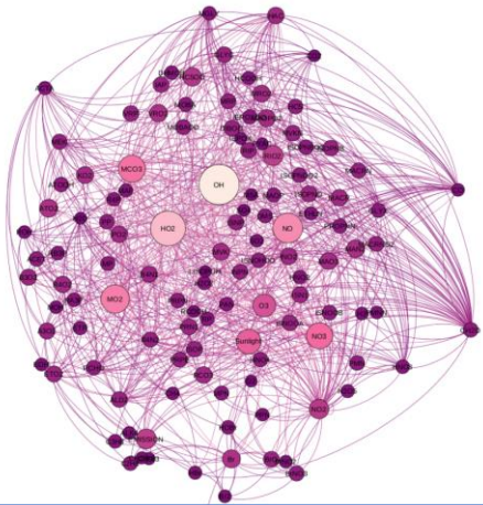
GEOS - Chem
