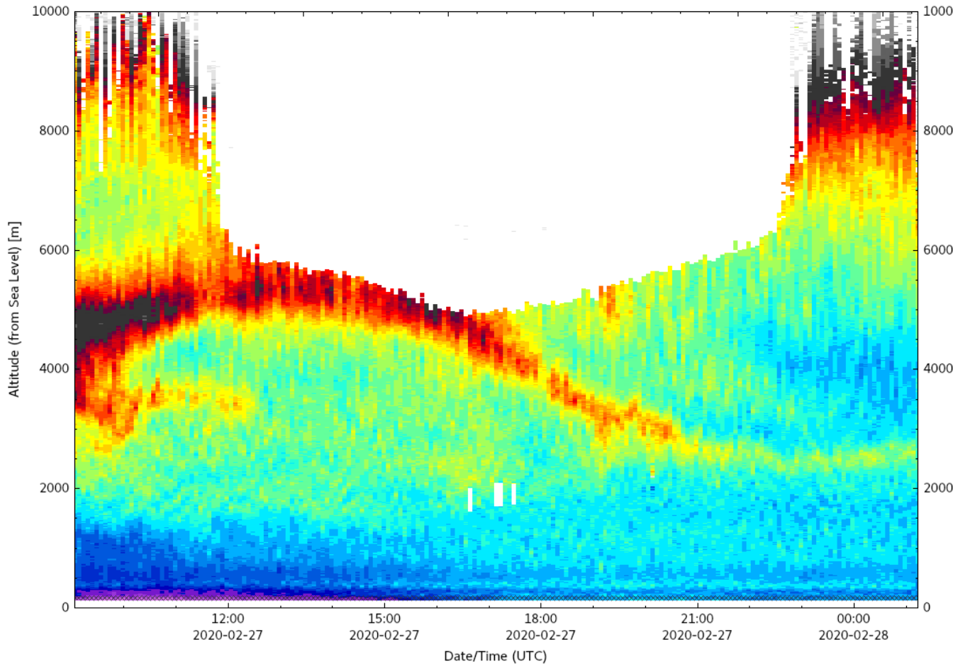
LMOL LaRC 2020-02-27 Level 1
