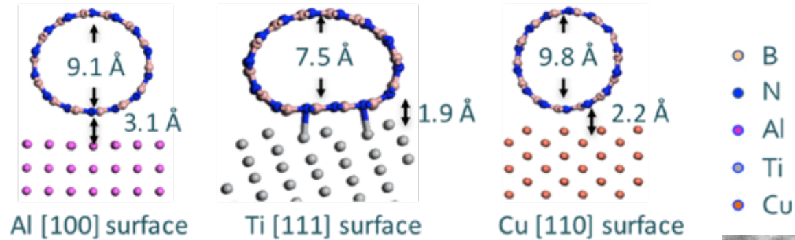
Pristine BNNT (7, 7)
