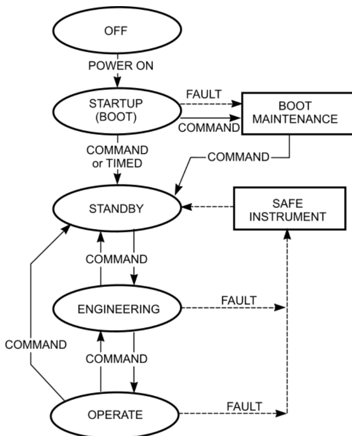
Fig. 15. Software Modes.
