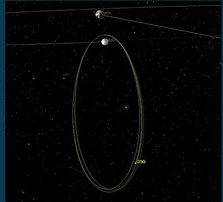
Ground tracking sim. parameters
