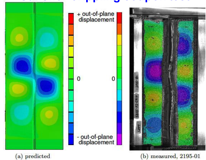
Stiffener crippling coupon test
