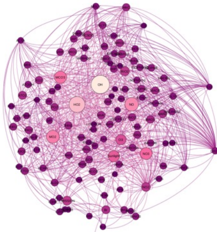
GEOS - Chem
