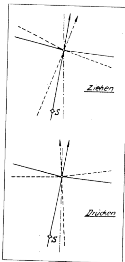
Fig. 19: Longitudinal control
