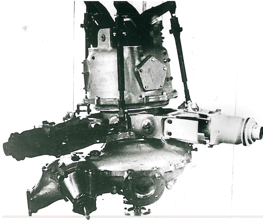
Fig. 22: Rotor hub
