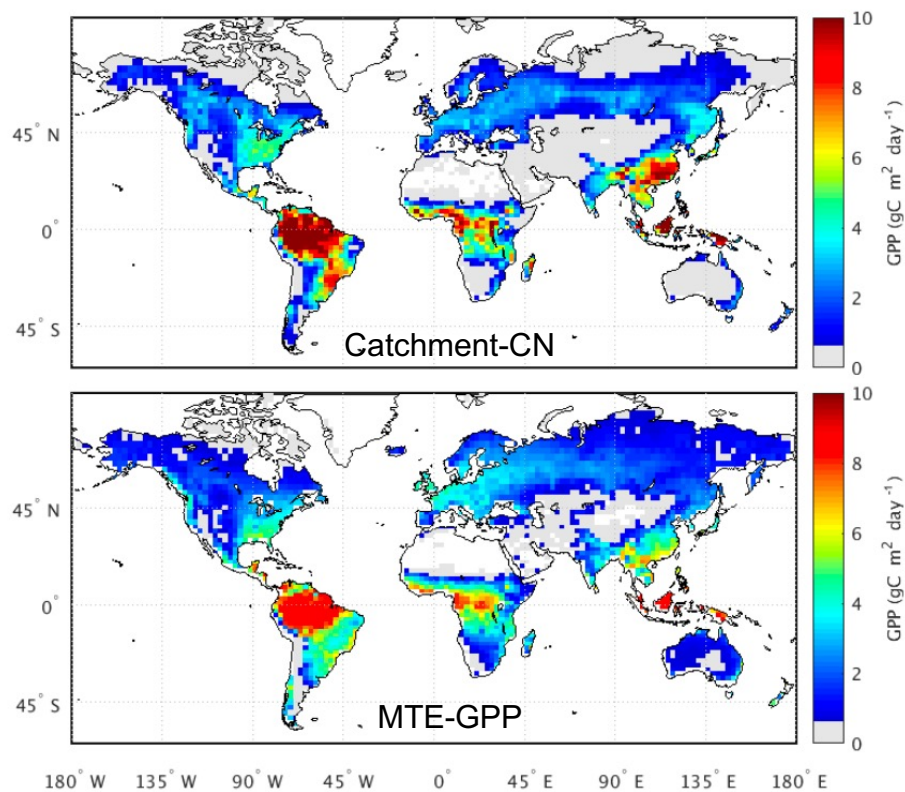
Lee et al. (2018) Biogeosci.
