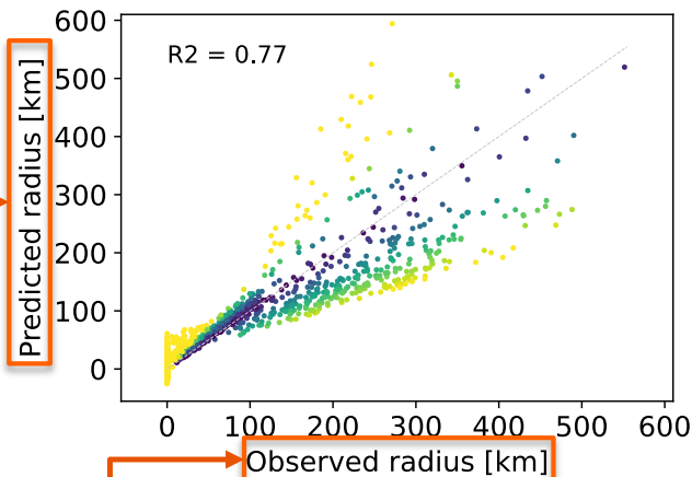
4. Gradient boosting
