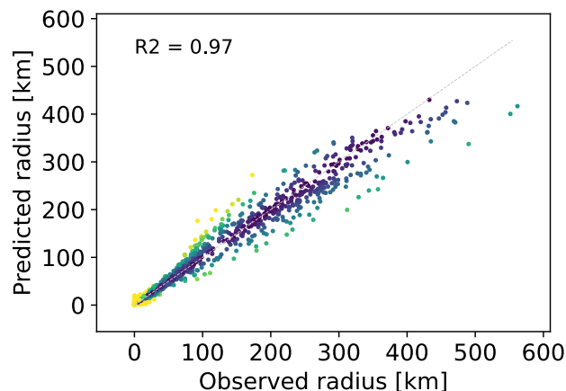
4. Gradient boosting
