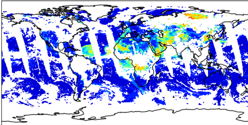
VIIRS SNPP NNR 550 nm AOD 20130802
