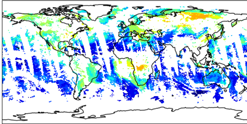
MODIS Aqua NNR 440-870 AE 20130802
