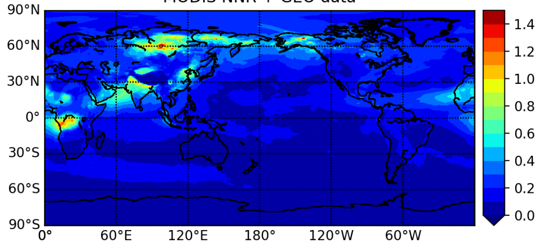
MODIS NNR + GEO data
