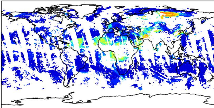
MODIS Aqua NNR 550 nm AOD 20130802
