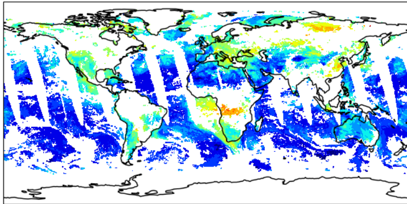
VIIRS SNPP NNR 440-870 AE 20130802
