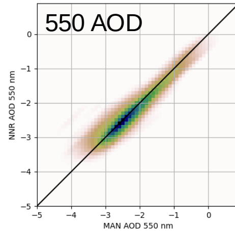
MODIS TERRA
