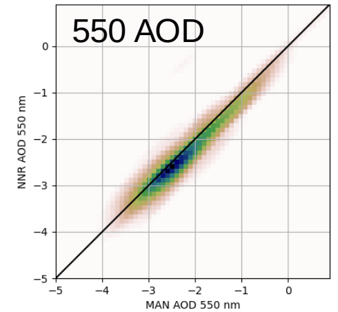
VIIRS SNPP
