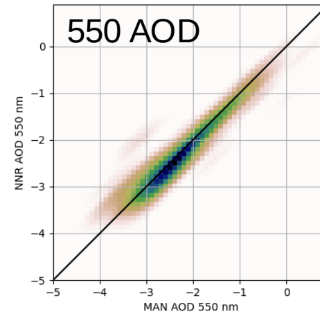
MODIS AQUA
