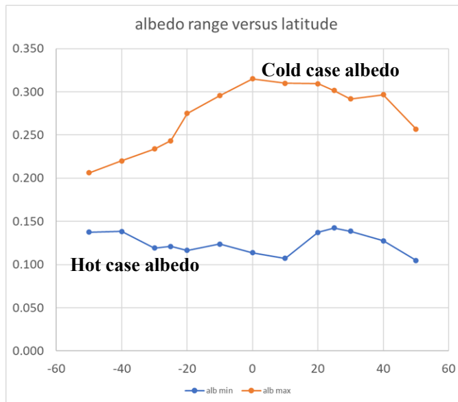
Max/min albedo vs latitude
