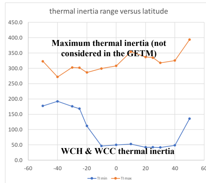
Max/min thermal inertia vs latitude
