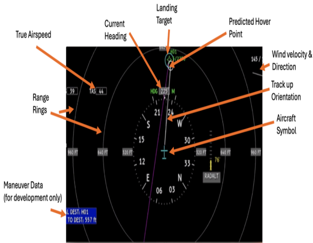
Fig. 9. Map/Navigation Display
