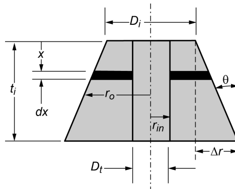
Figure F.3.—Frustum.
