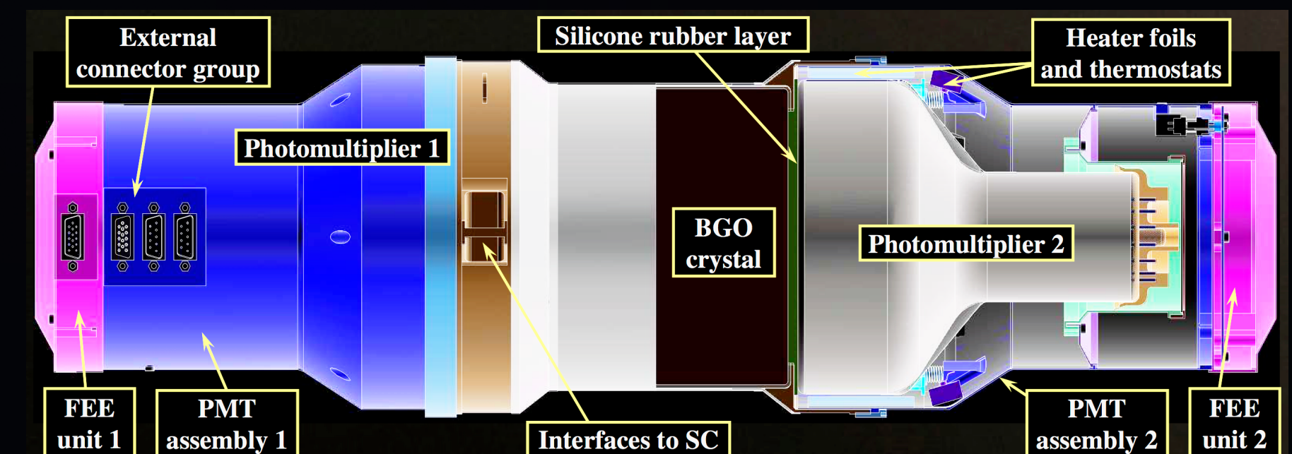
BGO Detector
