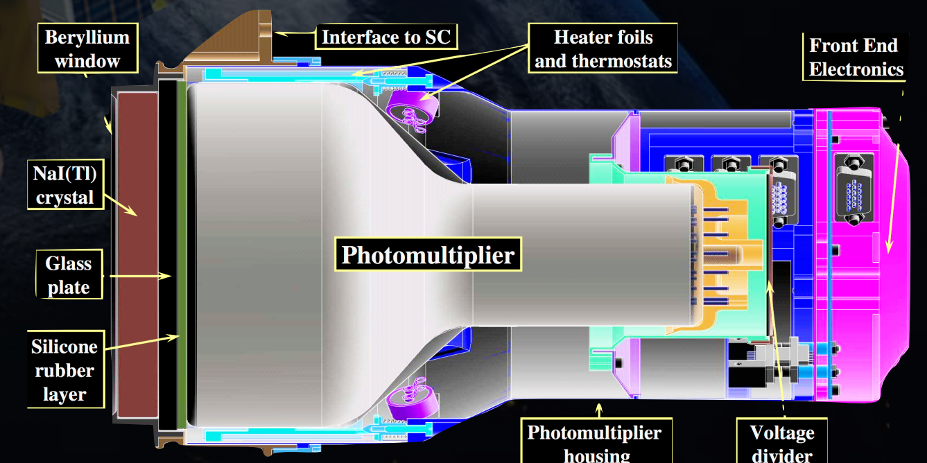
NaI Detector
