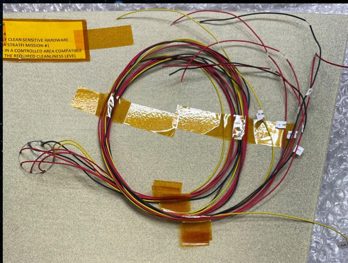
Flank Tile
